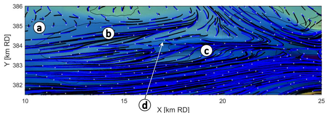
Figuur 3.12 Sedimenttransportpaden aan de zuidkant van de Vlake van de Raan op basis van modelberekeningen met golven (zwarte lijnen) en zonder golven (blauwe lijnen).
