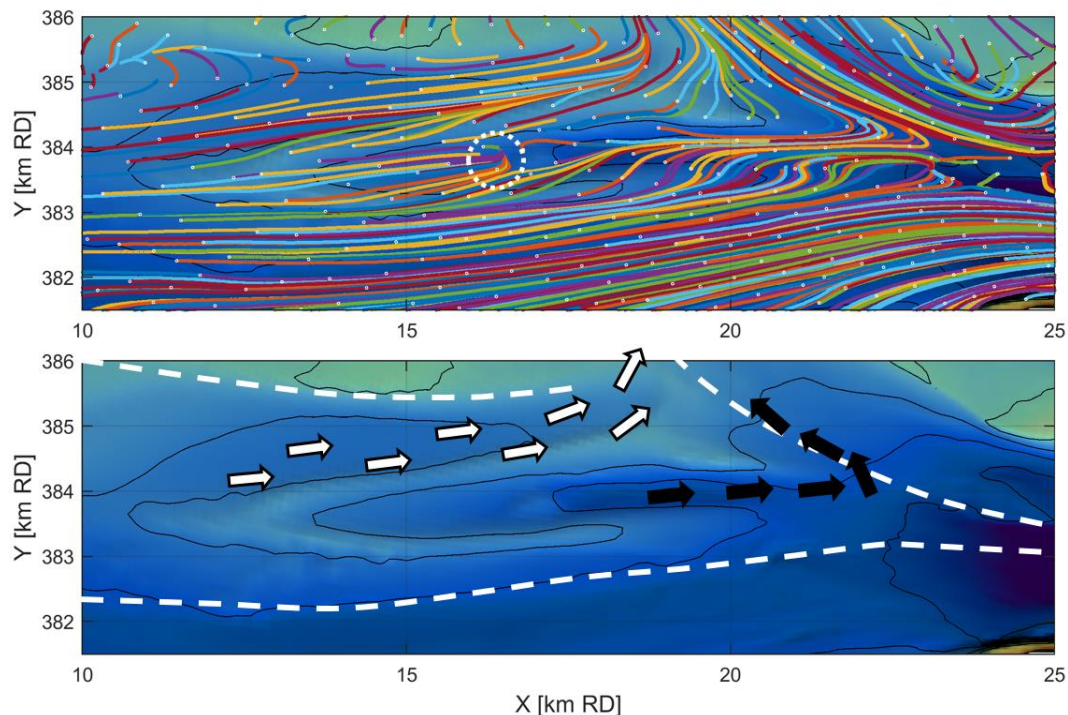
Figuur 3.6 Sedimenttransportpaden aan de zuidkant van de Vlake van de Raan. In het onderste paneel is een conceptuele beschrijving van de gemiddelde sedimenttransporten opgenomen die wordt toegelicht in de tekst.
