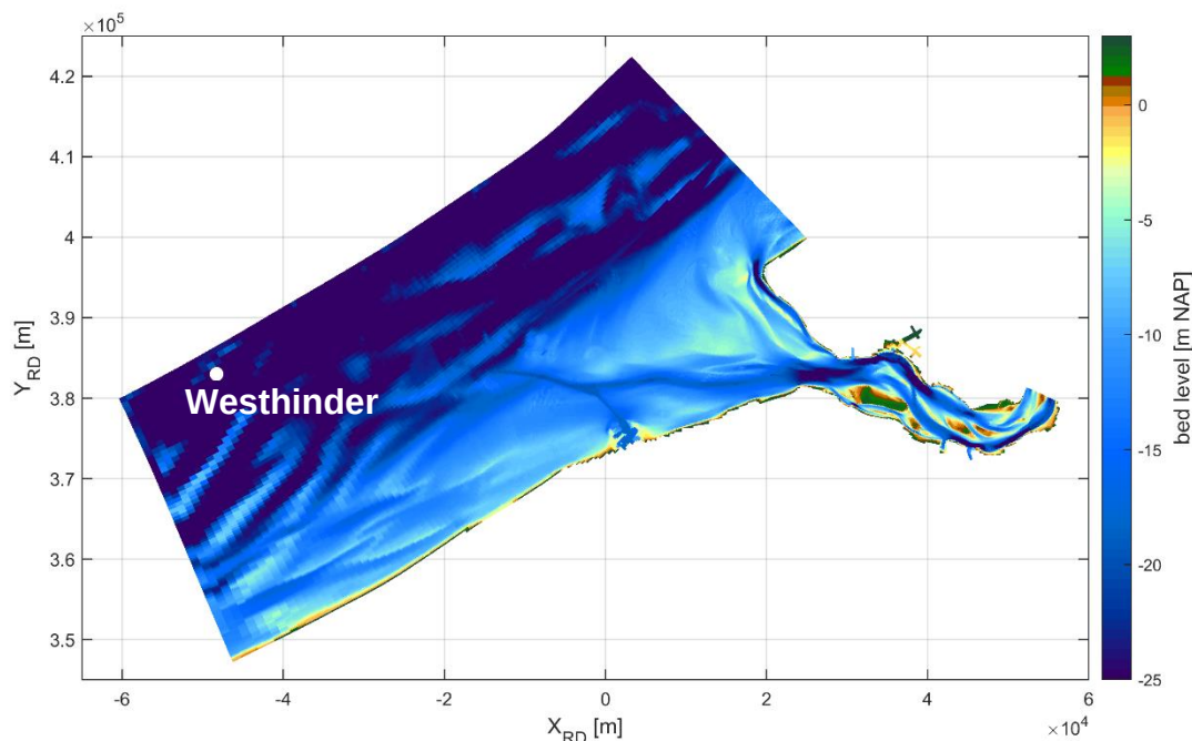
Figuur 2.1 Modeldomein van het Delft3D model dat in deze studie wordt toegepast. De kleurenschaal toont de bodemligging in het model. De bodemhoogte is gebaseerd op Vaklodgingen uit 2017. De randvoorwaarde voor golven is gebaseerd op gemeten golven bij Westhinder.
